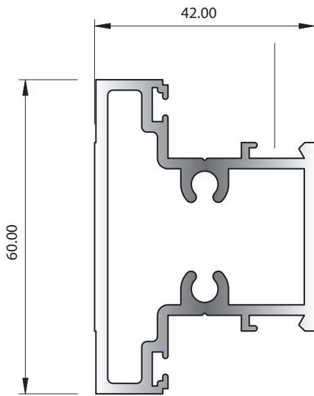
SECTION No. G251 1.400 kg/m P = 484.40
